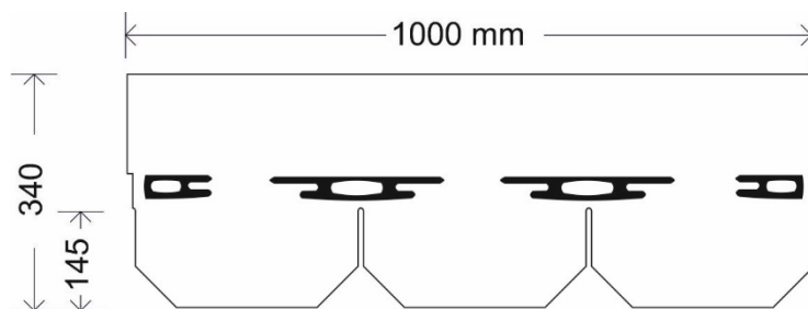
Fig. 1 - Dimensioni tegola Liberty
